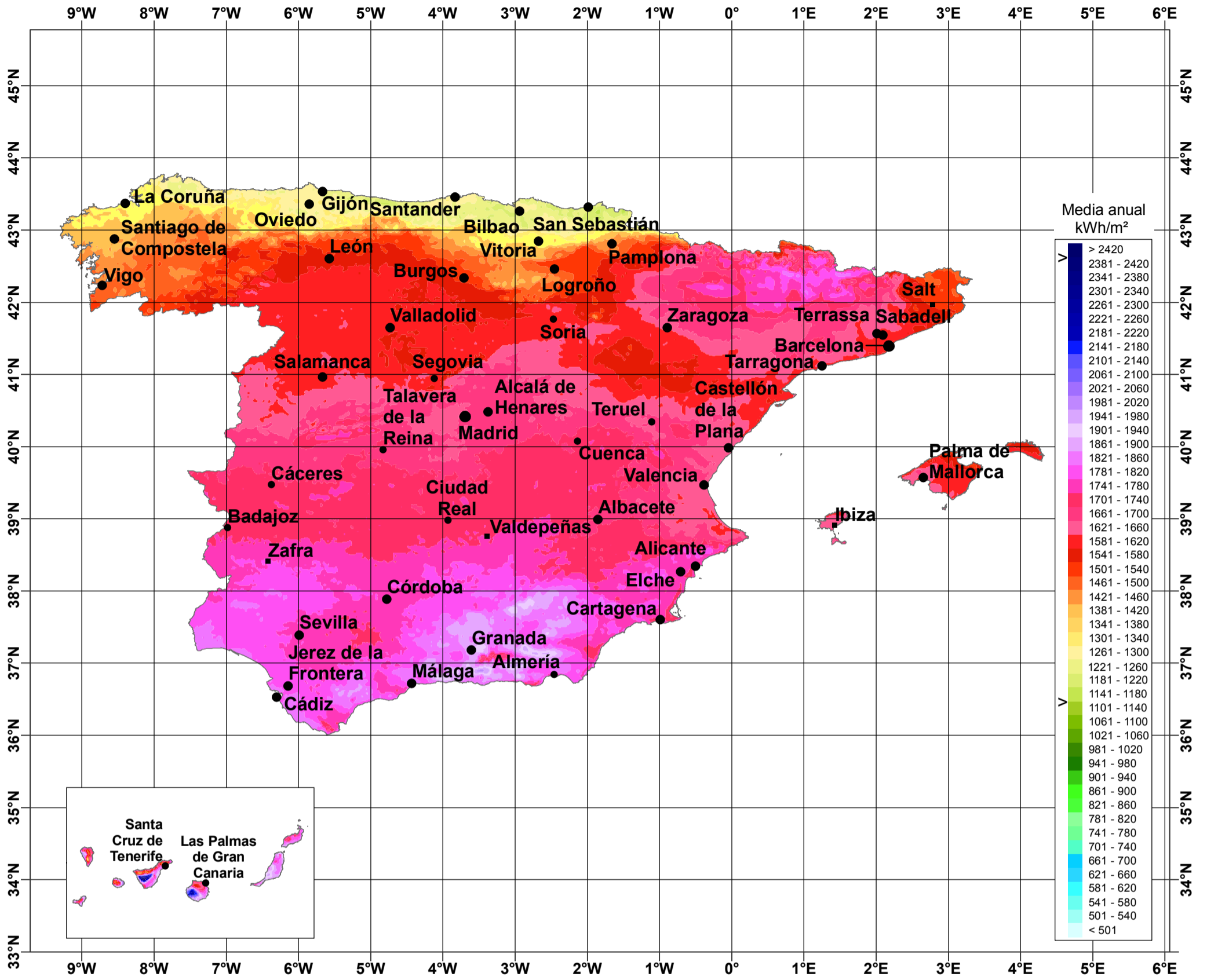
Strahlungskarte Spanien Daten: langjähriges Mittel Quelle: METEOTEST Produktion: 7.4.2008/fd
