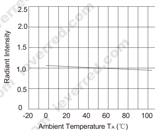
Fig.4 环境温度VS. 相对亮度
